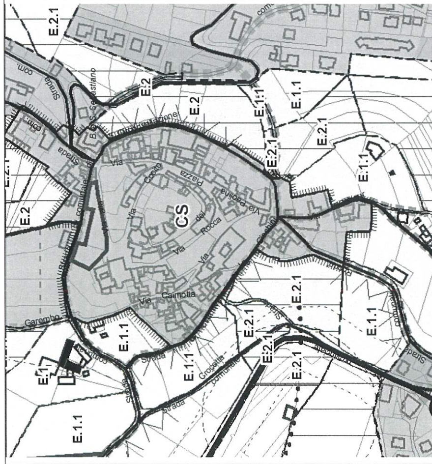
P2. assetto generale (sud) in scala originale 1:5.000- vigente
